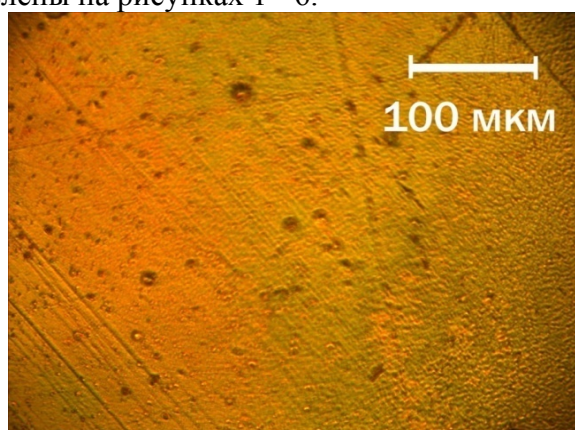
Рис. 2. Микрофотография облученной YBCO пленки при импульсной энергии 36 мДж и плотности мощности 8,1 \cdot 10^6 Вт/см 2 .
