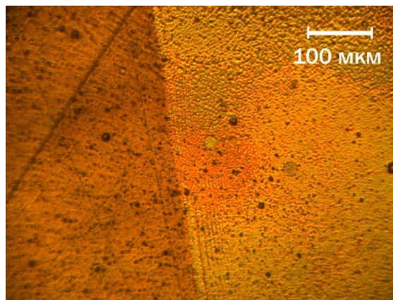
Рис. 4. Микрофотография облученной YBCO пленки при импульсной энергии 66 мДж и плотности мощности 1,5 \cdot 10^7 Вт/см 2 .
