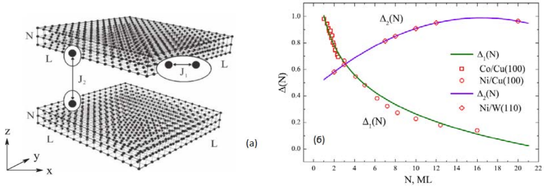
Рис. 1. Модель (а) мультислойной структуры, состоящей из двух ферромагнитных пленок, разделенных пленкой немагнитного металла. N, L – линейные размеры пленок; зависимость параметров анизотропии \Delta_1(N) и \Delta_2(N) от толщины пленки N в МС (б).
