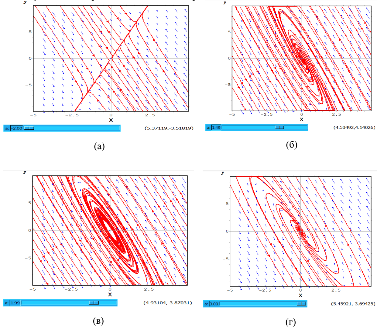
Рис. 1. Фазовые портреты в Maxima при изменении параметра a : неустойчивое седло (а), устойчивый фокус (б), центр (в), неустойчивый фокус (г)
