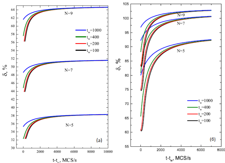
Рис. 2. Временная зависимость магнитосопротивления \delta(t, t_w) в структурах (а) Co/Cu/Co и (б) Pt/Co/Cu/Co/Pt с толщинами пленок Co N=5 - 9 МС при температурах T=T_c(N)/4 для времен ожидания t_w=100, 200, 400, 1000 MCS/s при эволюции из низкотемпературного начального состояния.
