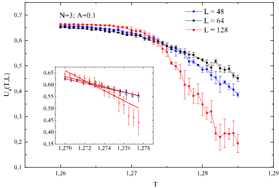
Рис. 1. Зависимость кумулянта Биндера U_4(T, L) с толщинами пленок N_1 = N_2 = 3ML . На вставке представлена линейная аппроксимация U_4(T, L) . Центр тяжести треугольника образованного пересечением линий соответствует критической температуре T_c = 1.273(2) .
