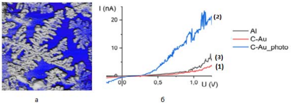
Рис. 1. Экспериментальные результаты исследования пленки Au с фрактальным дендритным характером при величине гранулы 20 нм: АСМ изображение (а) Вольтамперные характеристики: 1 – пленка, 2 – пленка при облучении, 3 - подложка (б)
