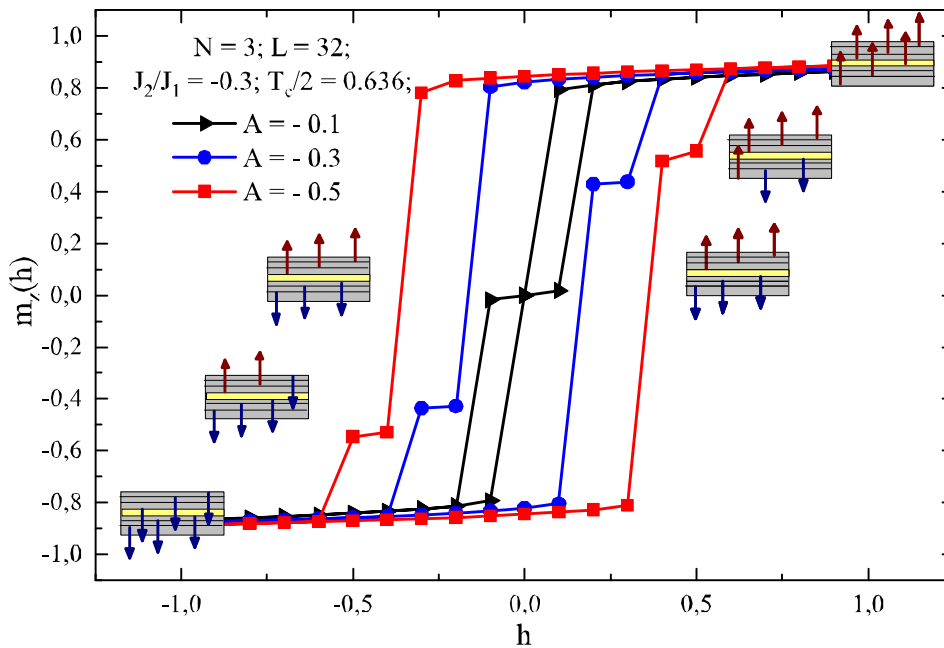
Рис. 2. Зависимость проекции намагниченности m_z(h) от внешнего поля h для случая межслоевого обменного взаимодействия J_2 = -0.3 с различными значениями константы одноионной анизотропии A = -0.1, -0.3, -0.5 при температуре T = T_c / 2 .
