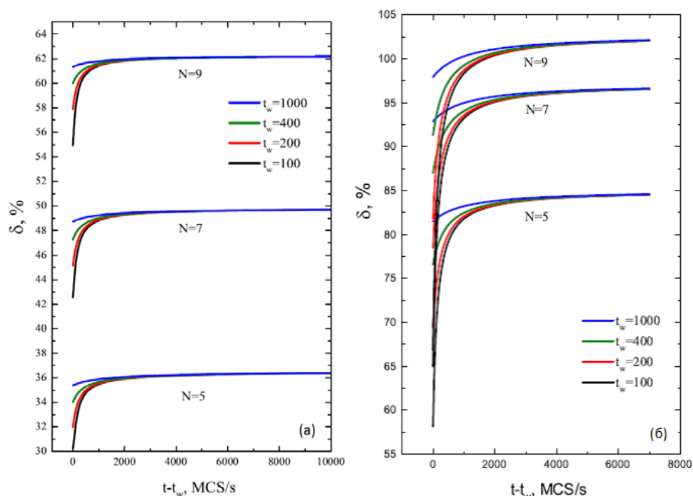
Рис. 3. Временная зависимость магнитосопротивления \delta(t, t_w) в структурах (а) Co/Cu/Co и (б) Pt/Co/Cu/Co/Pt с толщинами пленок Co N=5 - 9 МС при температурах T=T_c(N)/4 для времен ожидания t_w=100, 200, 400, 1000 MCS/s при эволюции из высокотемпературного начального состояния.
