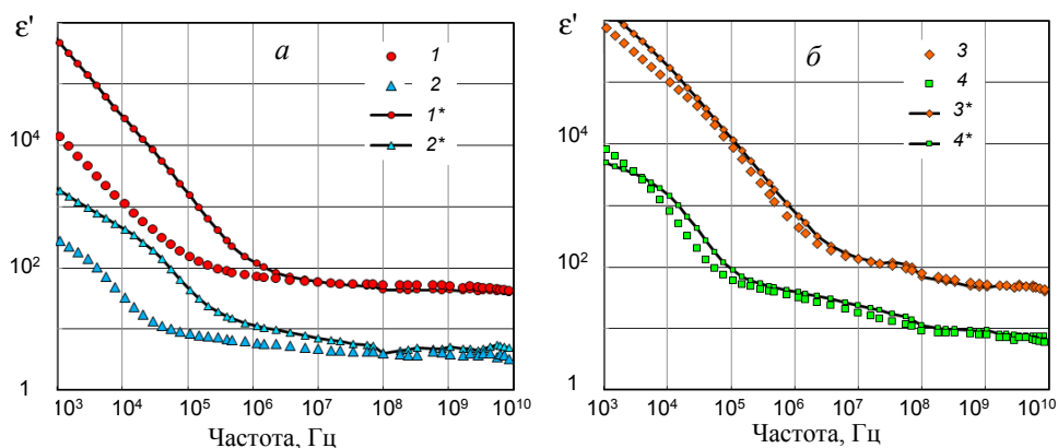
Рис. 3. Частотные зависимости действительной части КДП для (а) каолина; (б) бентонитовой глины Са-формы, полностью насыщенных 1, 2, 3, 4 – дистиллированной водой; 1*, 2*, 3*, 4* – солевым раствором NaCl концентрацией 17 г/л; 1, 1*, 3, 3* – при температуре +25^\circ\text{C} ; 2, 2*, 4, 4* – при температуре -15^\circ\text{C} .
