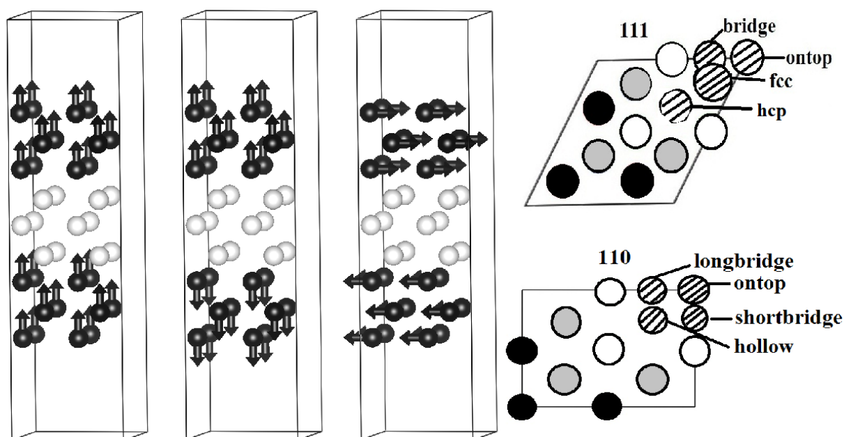
Рис. 1. Конфигурации атомов и направление спинов в суперячейке для трех атомных слоев кобальта с обеих сторон пластины меди.
