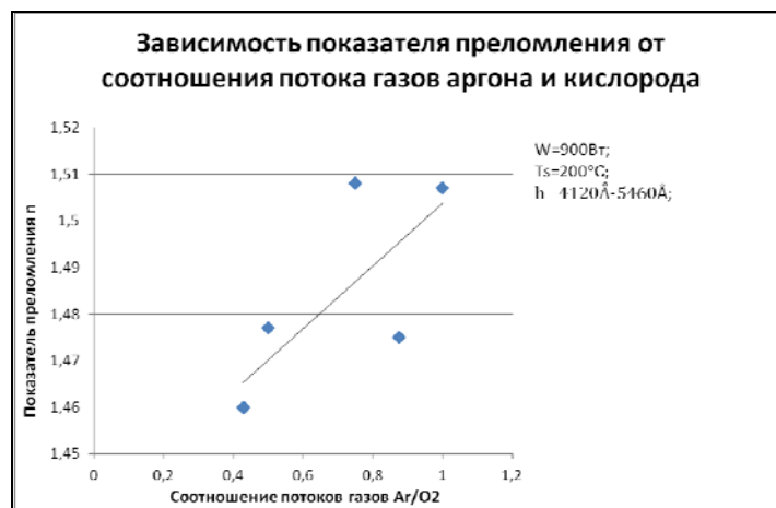
Рис. 3. Зависимость показателя преломления пленок SiO 2 от соотношения потоков аргона и кислорода.
