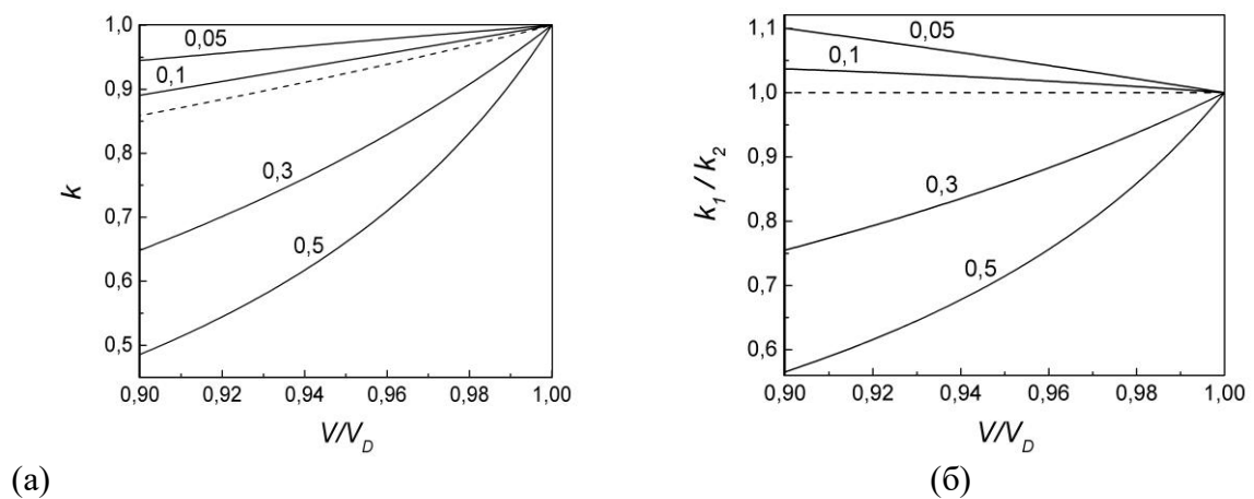
Рис. 1. Зависимость коэффициента распределения k от V/V_D ; k_e = 0,1 ; c_0 = ; V_D/V_{DI} = 1 ; \alpha_A = 1 ; \alpha_B = 0 ; V_D/V_0 = 0,05; 0,1; 0,3; 0,5 (значения показаны на кривых); (а) сплошные линии - коэффициент распределения k_1 согласно (8), пунктирная линия - k_2 согласно (1); (б) отношение коэффициентов k_1/k_2 .
