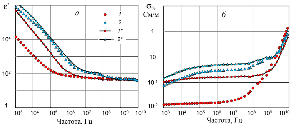
Рис. 1. Частотные зависимости действительной части КДП (а) и удельной эквивалентной проводимости (б) при температуре +25°C 1, 1* – каолина; 2, 2* – бентонитовой глины Са-формы. 1, 2 – насыщение дистиллированной водой, 1*, 2* – насыщение солевым раствором NaCl концентрацией 17 г/л.
