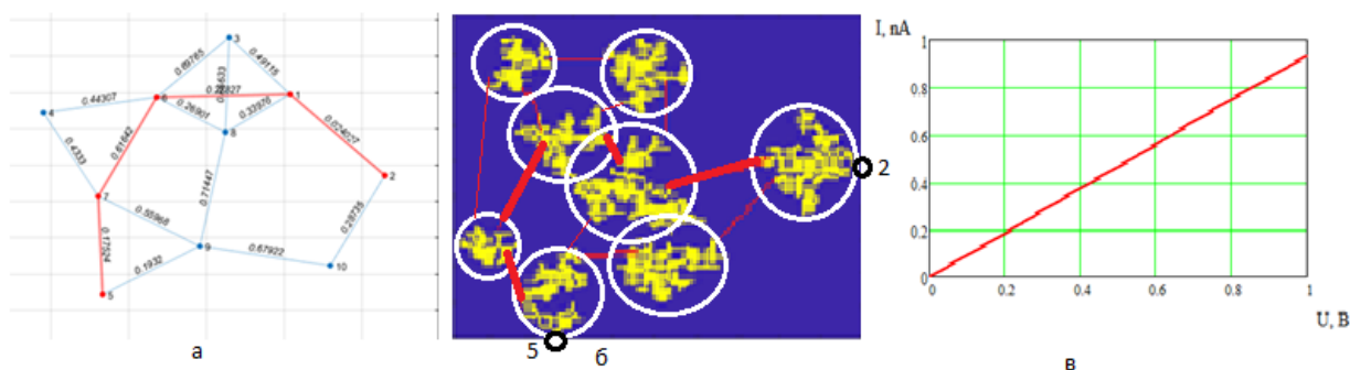
Рис. 2. Результаты моделирования: случайный граф (б), DLA модель островковой пленки при вероятности слипания и вязкости 0.2, с дорожками проводимости между островками и сферами покрытия кластеров, расчетная туннельная ВАХ Au пленки.
