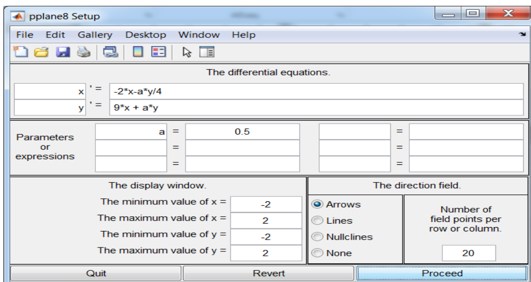
Рис. 2. Интерфейс программы PPLANE8 для системы второго порядка
