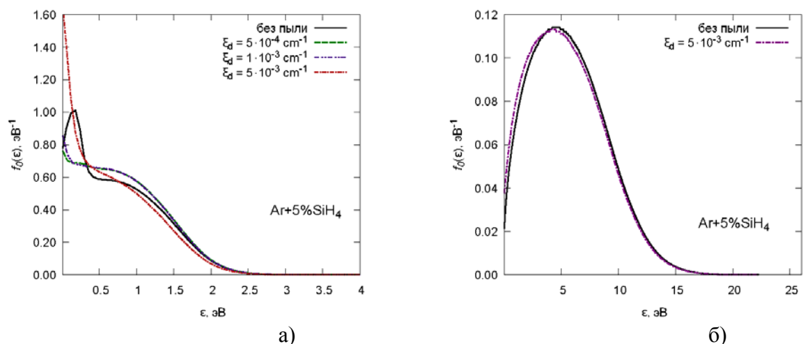
Рис. 1. ФРЭЭ в смеси Ar+5%SiH 4 при наличии частиц пыли а) E/N=5 \cdot 10^{-17} \text{ В} \cdot \text{см}^2 ; б) E/N=10^{-15} \text{ В} \cdot \text{см}^2
