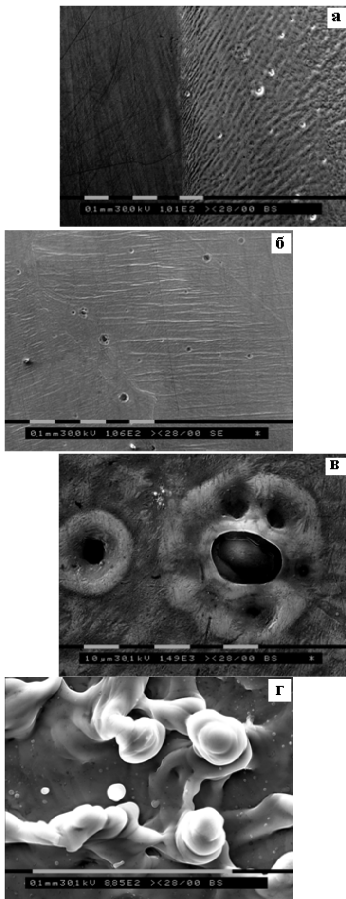
Рис.2. Морфология поверхности магния, облученного с плотностью тока 100 \text{ A/cm}^2 (а, б) и 150 \text{ A/cm}^2 (в, г)
