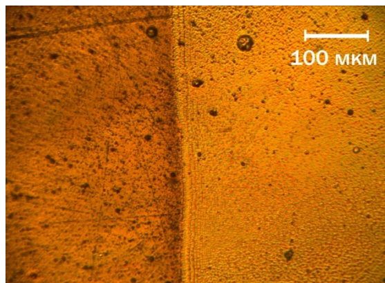
Рис. 6. Микрофотография облученной YBCO пленки при импульсной энергии 120 мДж и плотности мощности 2,7 \cdot 10^7 Вт/см 2 .
