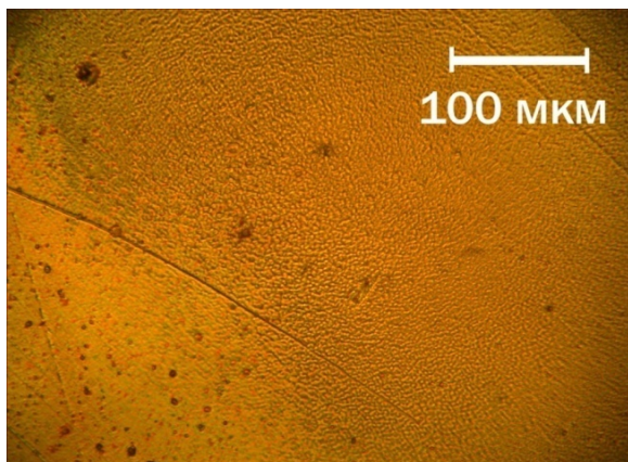
Рис. 3. Микрофотография облученной YBCO пленки при импульсной энергии 54 мДж и плотности мощности 1,2 \cdot 10^7 Вт/см 2 .
