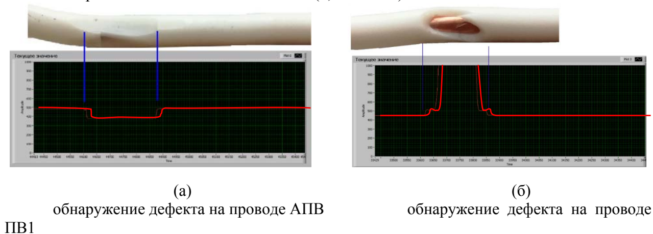
Рис. 2. Графики изменения погонной емкости
