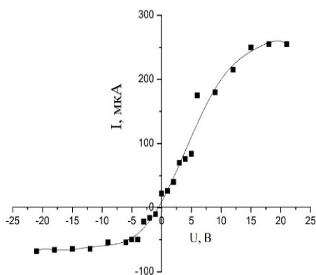
Рис.2. ВАХ зонда Ленгмюра в факеле лазерной плазмы мишени YBCO.
