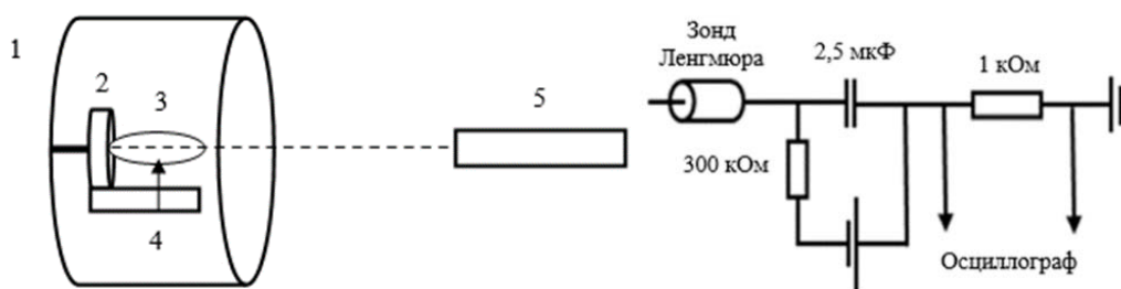
Рис.1. Вакуумная установка для изучения лазерной плазмы и электрическая эквивалентная схема подключения зонда Ленгмюра.
