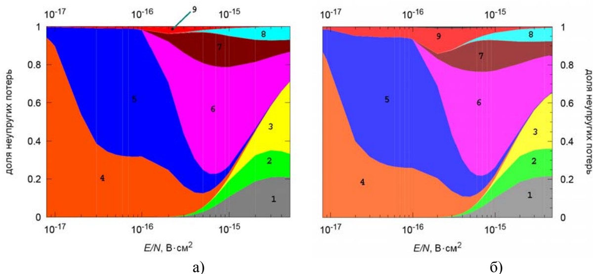
Рис.4 Распределение потерь энергии в неупругих столкновениях в плазме Ar+5%SiH 4 при пылесодержании а) \xi_d = 1 \cdot 10^{-3} см -1 , б) \xi_d = 5 \cdot 10^{-3} см -1 . Ar: 1 – возбуждение метастабильных уровней 3 P 0 , 3 P 2 ; 2 – полное возбуждение; 3 – ионизация. SiH 4 : 4 – колебательное возбуждение моды \nu_{24} ; 5 – колебательное возбуждение моды \nu_{13} ; 6, 7 – электронное возбуждение; 8 – ионизация, 9 – прилипание к пыли
