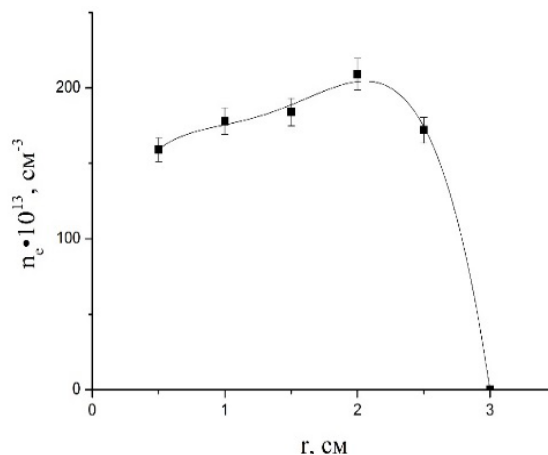
Рис.5. Зависимость концентрации электронов от расстояния зонд-мишень.
