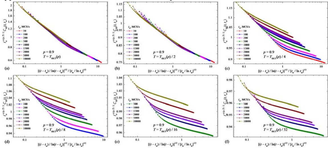
Рис. 3. Динамические скейлинговые зависимости спин-спиновой автокорреляционной функции C(t, t_w) одновихревой неравновесной критической релаксации двумерной структурно неупорядоченной XY-модели. Спиновая концентрация p = 0.9 . Температуры замораживания системы T \leq T_{\text{вкт}}(p) .
