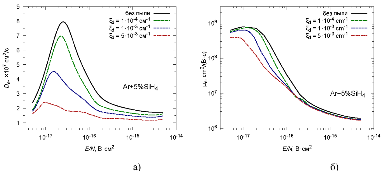
Рис. 2. Коэффициент а) диффузии; б) подвижности электронов в плазме Ar+5%SiH 4 при наличии частиц пыли
