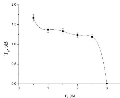
Рис.3. Зависимость электронной температуры от расстояния зонд-мишень.
