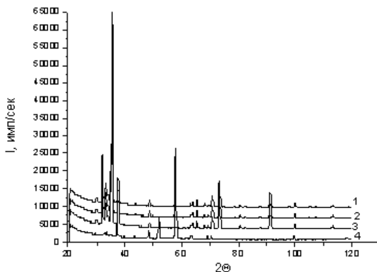
Рис. 1. Дифрактограммы магния до(1) и после облучения МИП с плотностью тока: 2-50, 3-100 и 4-150 А/см 2 одним импульсом
