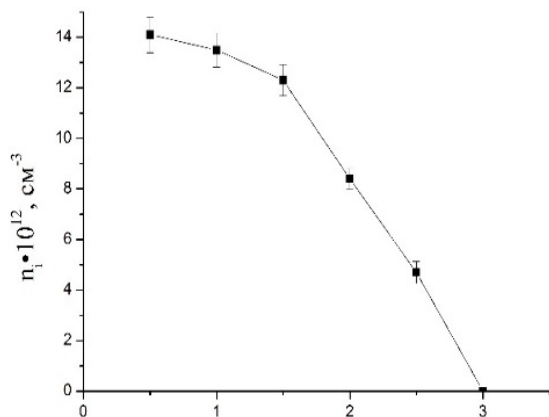
Рис.4. Зависимость концентрации ионов от расстояния зонд-мишень.
