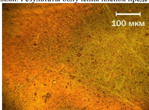
Рис. 1. Микрофотография облученной YBCO пленки при импульсной энергии 18 мДж и плотности мощности 4,0 \cdot 10^6 Вт/см 2 .
