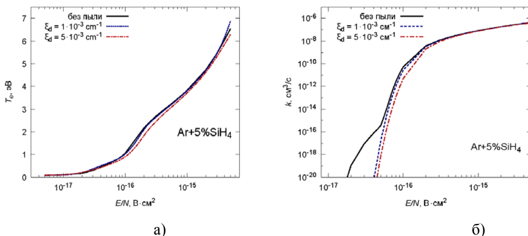
Рис 3. а) Температура электронов; б) константа скорости диссоциации молекул SiH 4 в плазме Ar+5%SiH 4 при наличии частиц пыли
