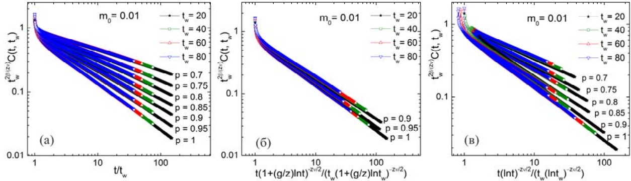
Рис. 1. Зависимости скейлинговых функций F_C(t/t_w) = t_w^{2\beta/(vz)} C(t, t_w) от t/t_w (а) и с учетом логарифмических поправок в виде F_C(t(1+(g/z)\ln t)^{z/2}/(t_w(1+(g/z)\ln t_w)^{z/2})) для системы p=0.95 (б) и в виде F_C(t \ln^{z/2} t/(t_w \ln^{z/2} t_w)) для систем с p \leq 0.9 (в) при эволюции из высокотемпературного начального состояния с намагненностью m_0 = 0.01 .
