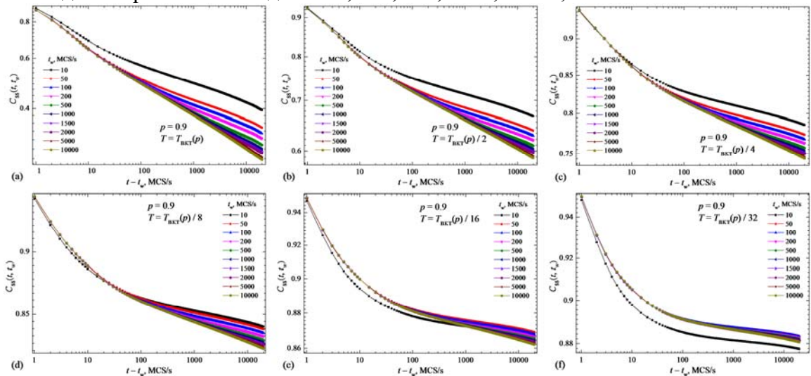
Рис. 2. Двухвременные динамические зависимости спин-спиновой автокорреляционной функции C(t, t_w) одновихревой неравновесной критической релаксации двумерной структурно неупорядоченной XY-модели. Спиновая концентрация p = 0.9 . Температуры замораживания системы T \leq T_{\text{ВКТ}}(p) .
