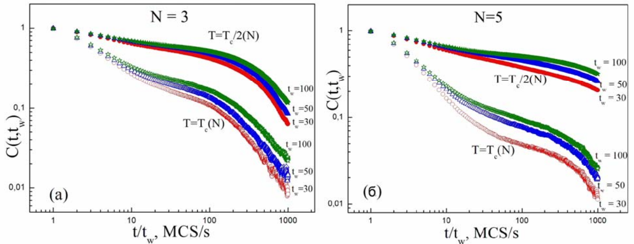
Рис. 2. Зависимость автокорреляционной функции при N=3 (а) и N=5 (б) от времени наблюдения при временах ожидания t_w=30;50;100 при T=T_c(2.9033) , и так же при T=T_c/2(1.4516) .
