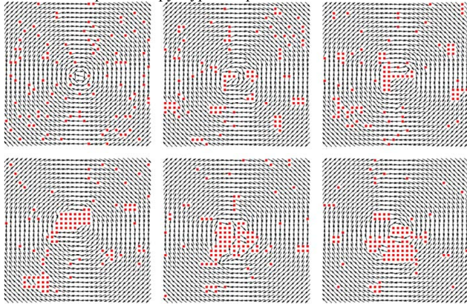
Рис. 1. Визуализация динамики отжига дефектов структуры вихрем в одновихревой неравновесной критической релаксации двумерной структурно неупорядоченной XY-модели. Времена наблюдения: 0, 100, 500, 2000, 10000, 20000 MCS/s.
