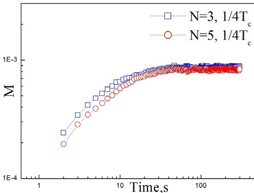
Рис. 1. Критическая эволюция шахматной намагниченности из высокотемпературного состояния.
