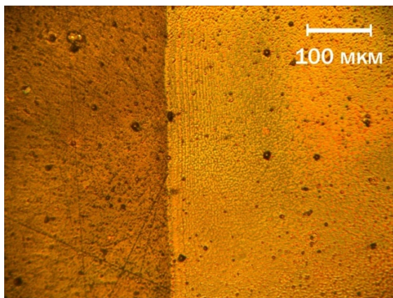
Рис. 5. Микрофотография облученной YBCO пленки при импульсной энергии 100 мДж и плотности мощности 2,2 \cdot 10^7 Вт/см 2 .
