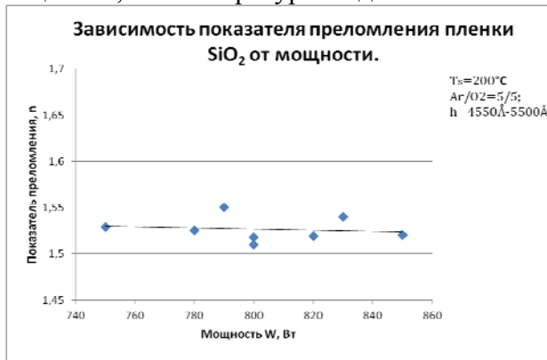
Рис. 1. Зависимость показателя преломления пленки \text{SiO}_2 от мощности.
