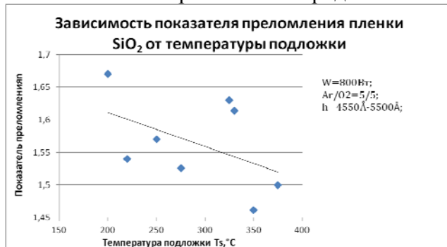
Рис. 2. Зависимость показателя преломления пленки \text{SiO}_2 от температуры подложки.
